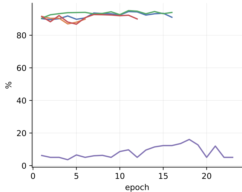
Source validation macro-F1
