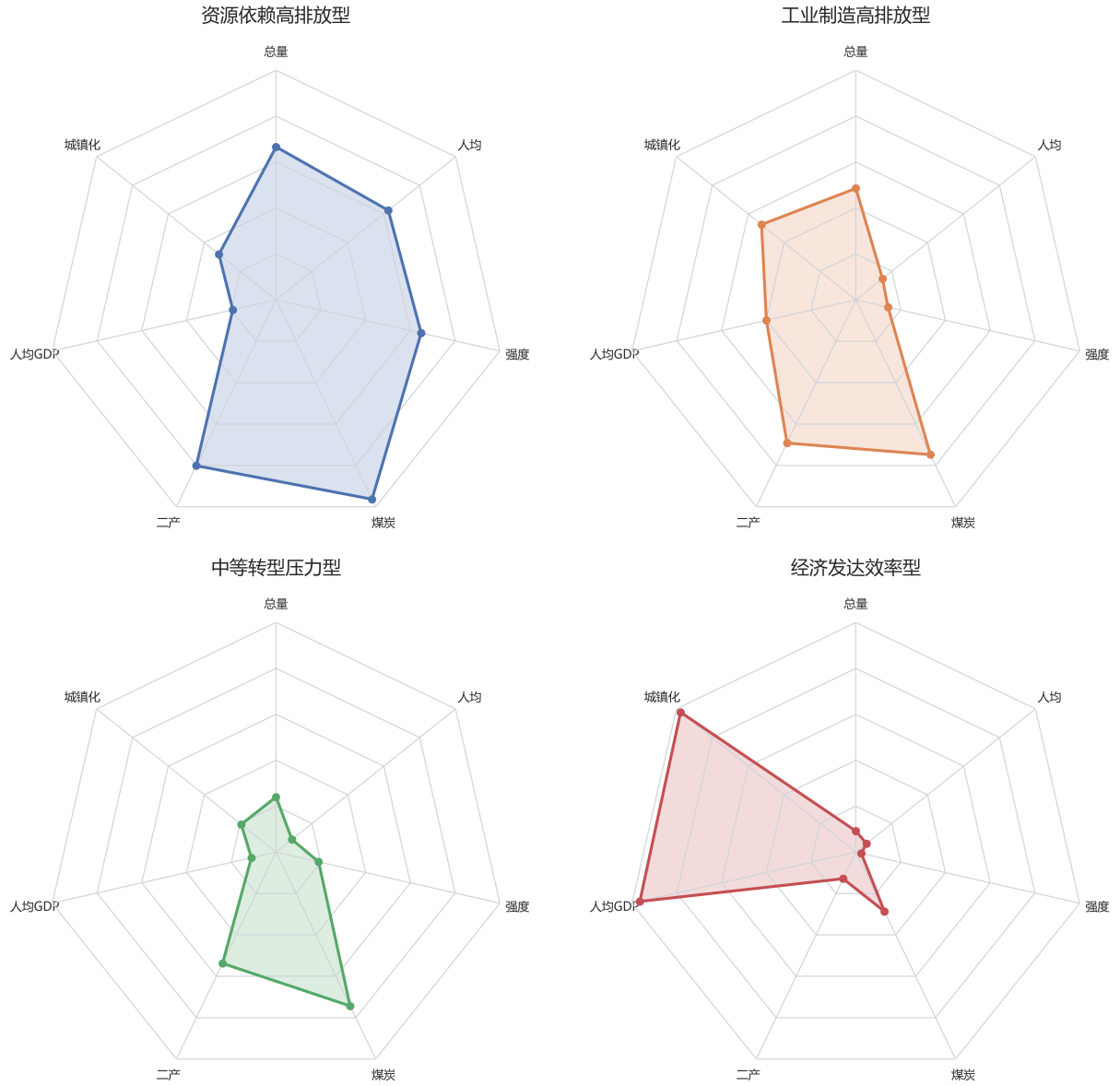
图 5 K-means 四类省份标准化均值画像雷达图
