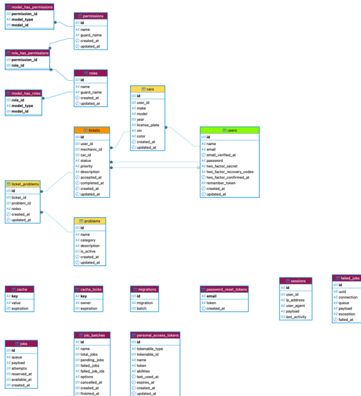
Figure 1: Az onlyfix alkalmazás adatbázisának ER diagramja
