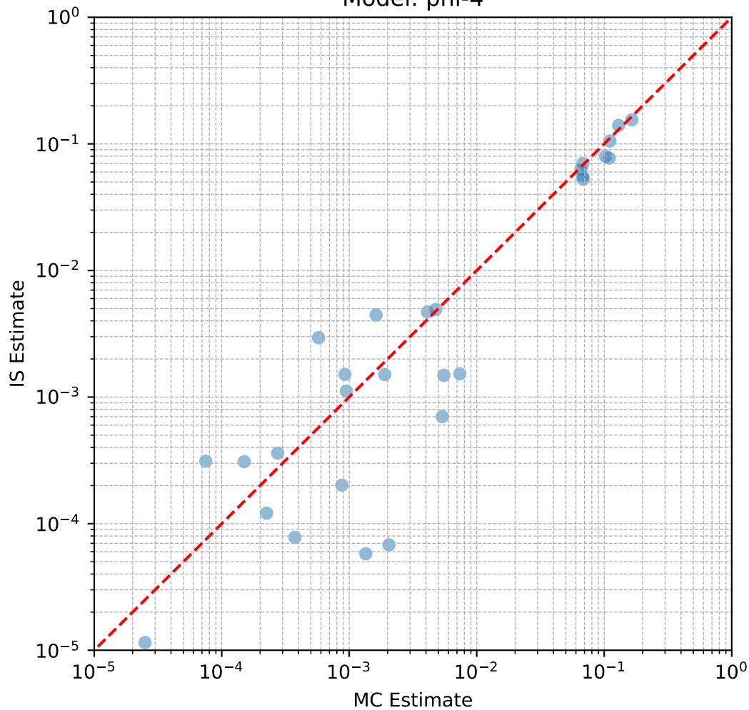
Model: phi-4
