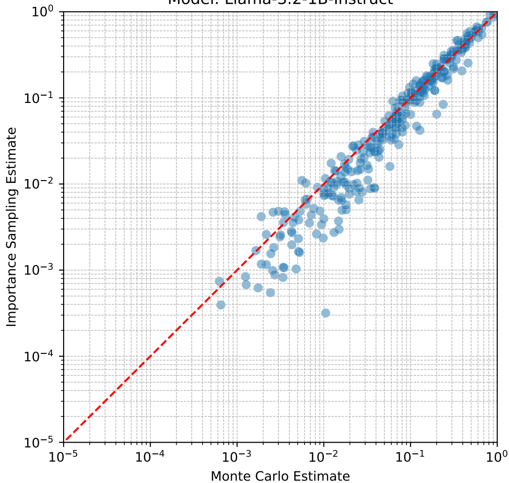
Model: Llama-3.2-1B-Instruct
