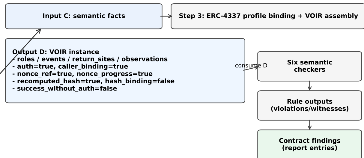
(d) Step 3 VOIR Assembly and Checker Consumption
