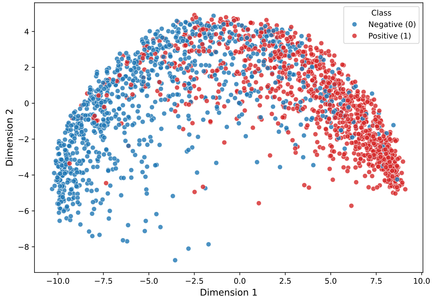
PCA of HMB-Net (h_k)
