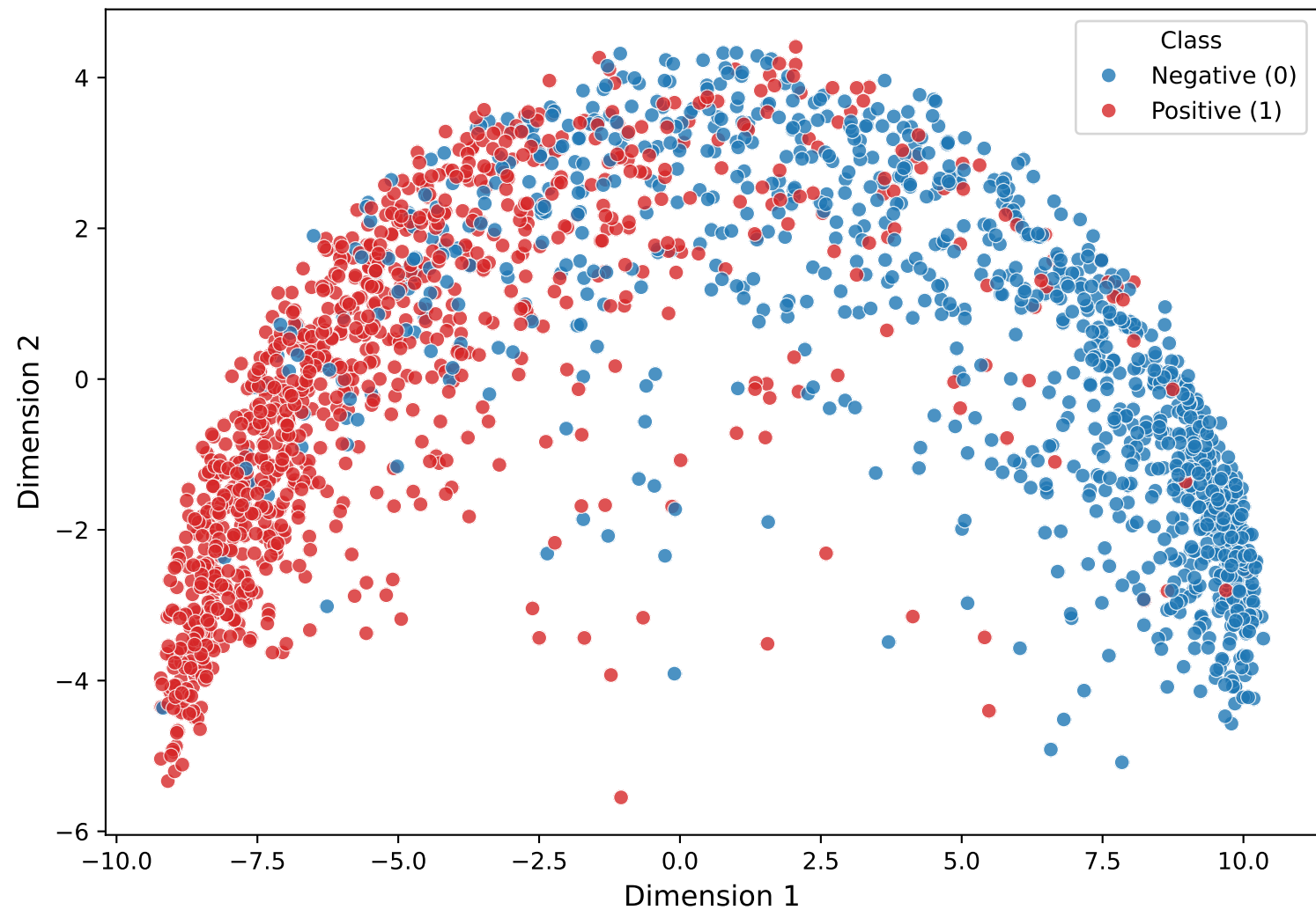
PCA of HMB-Net (r_k)
