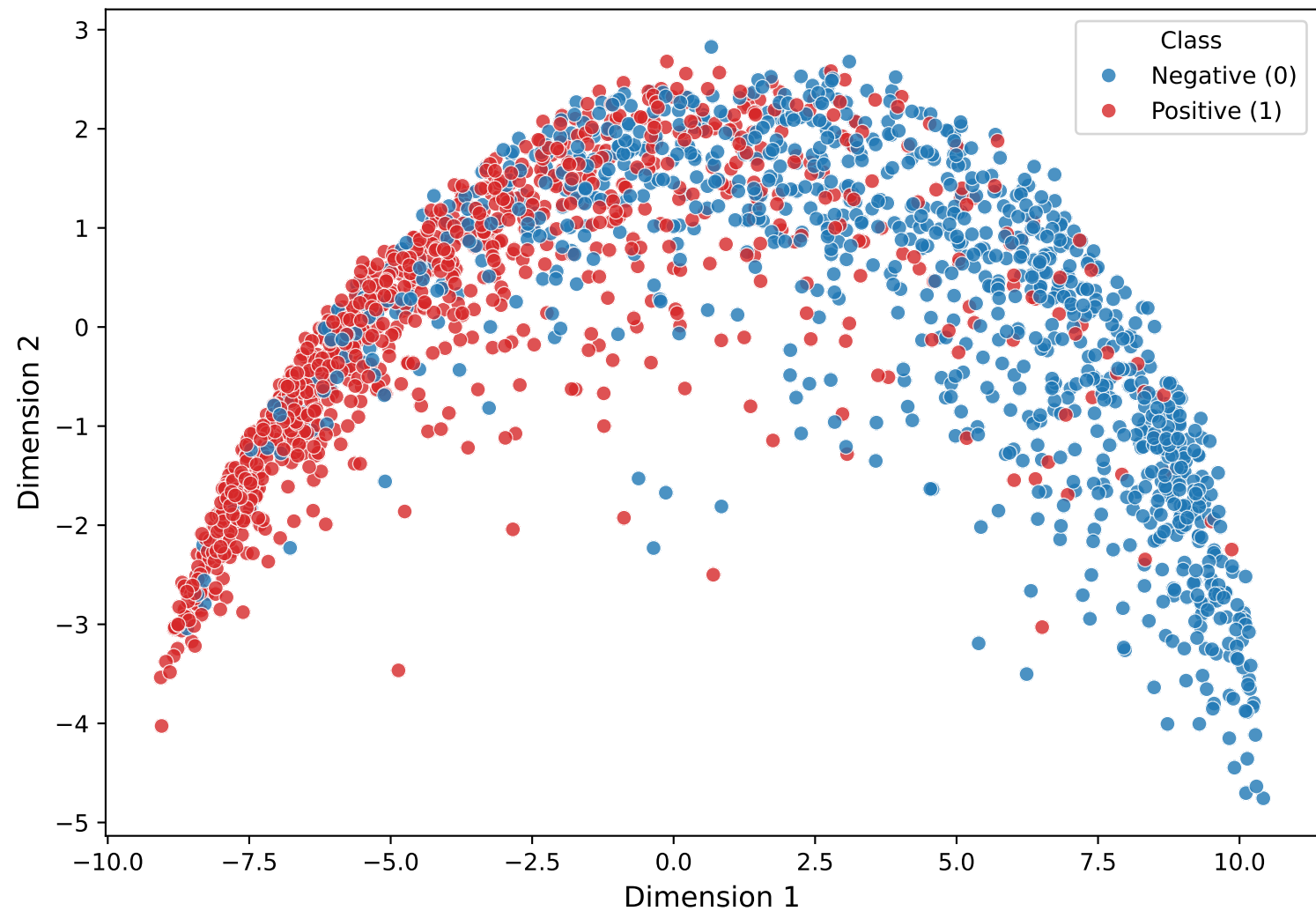
PCA of HMB-Net (r_l)
