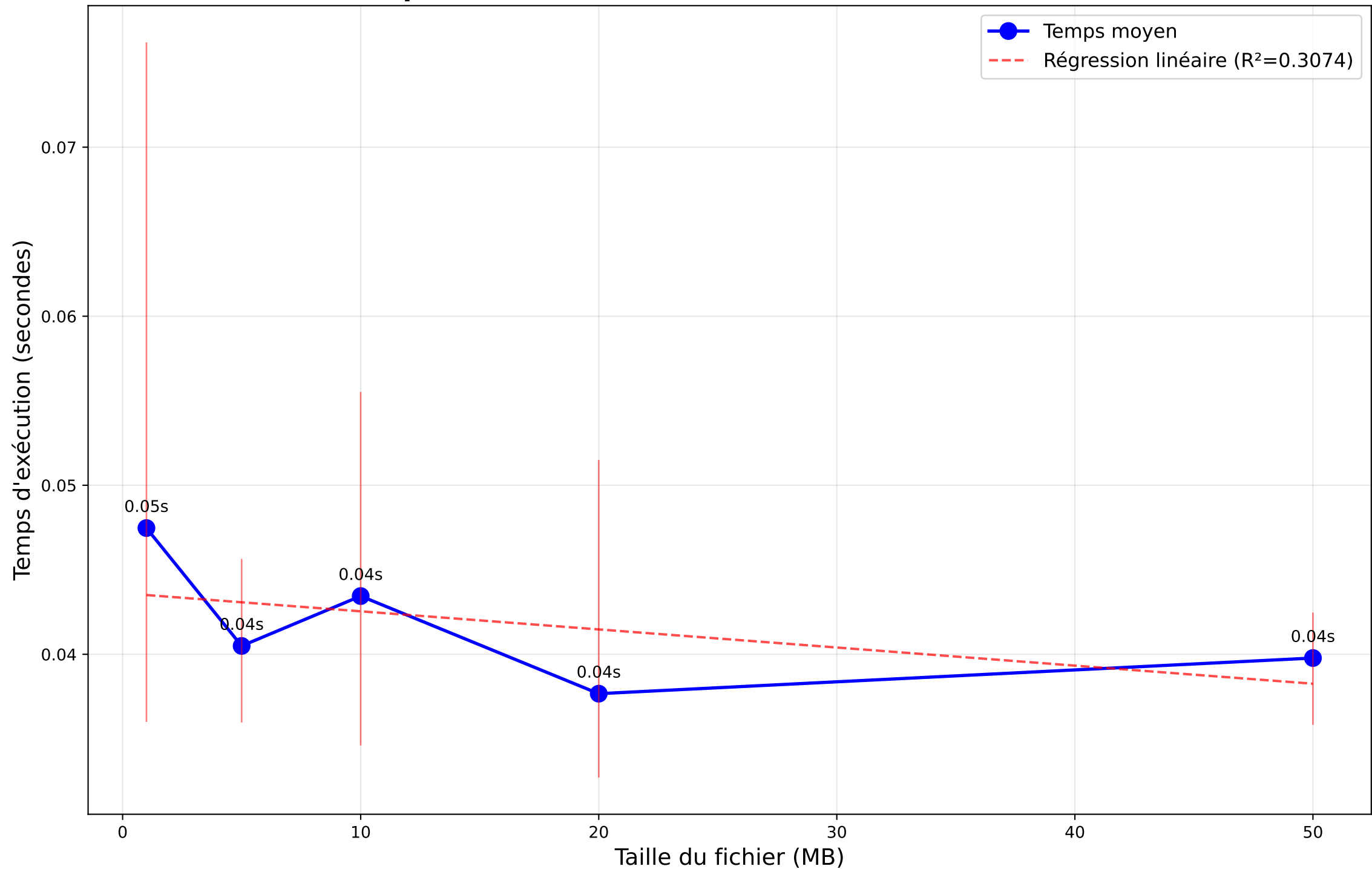
Temps d'exécution du Word Count vs Taille du fichier
