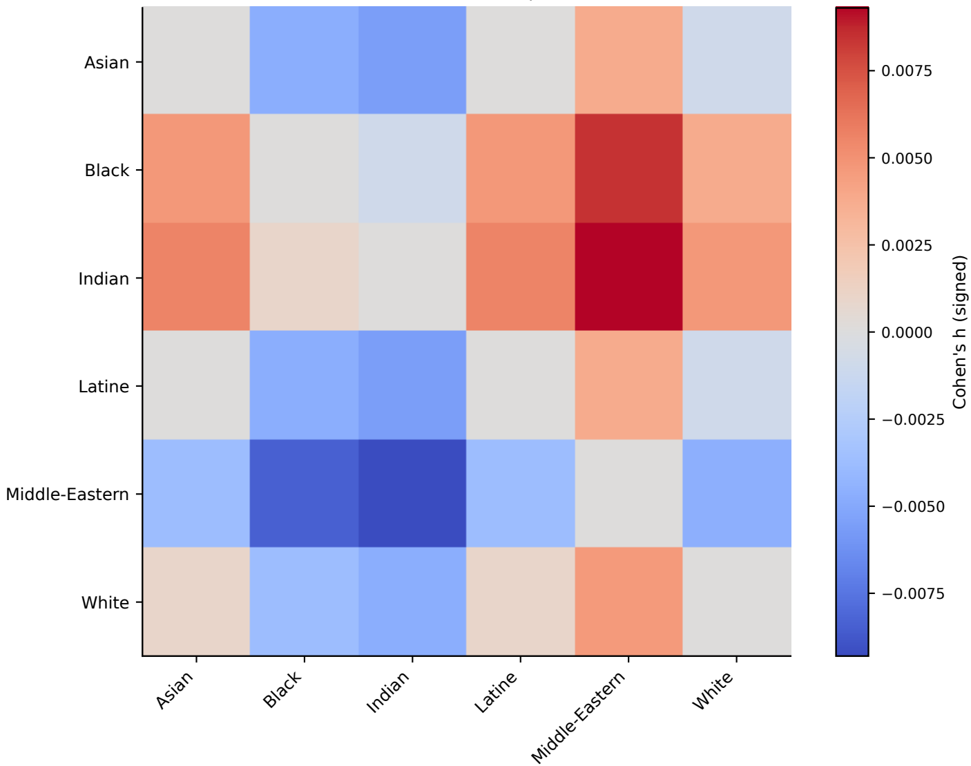
Effect size — trait pairs
