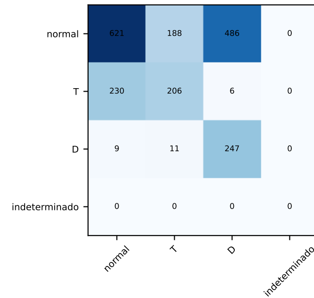
SVM
