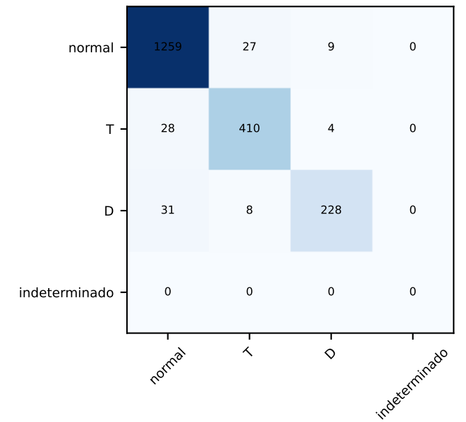
KNN_estend
