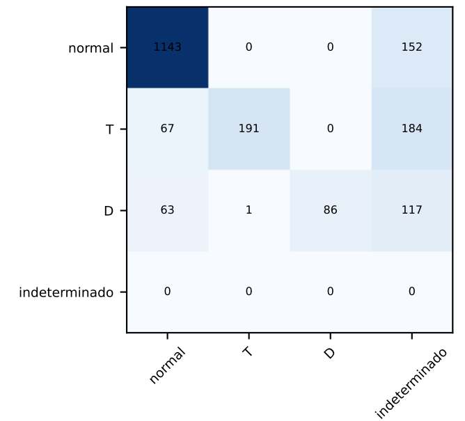
KNN
