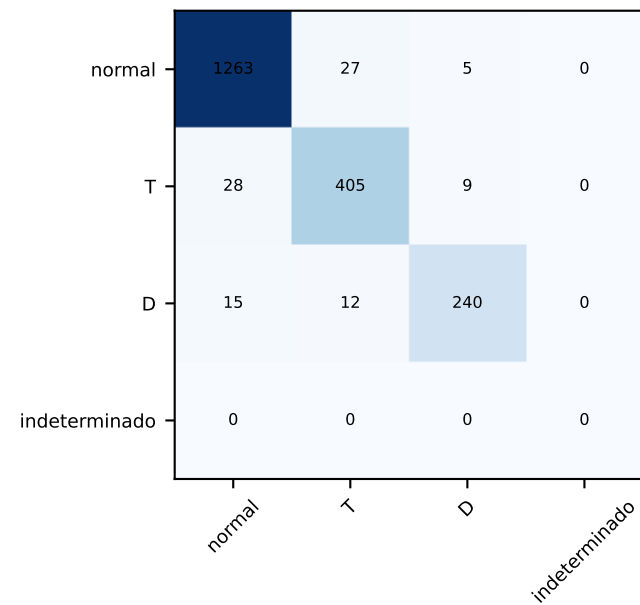
HistGB
