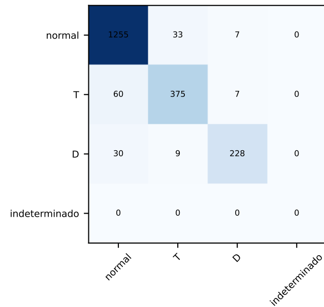
ANN
