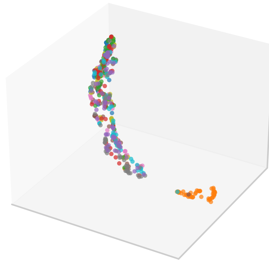
UMAP
