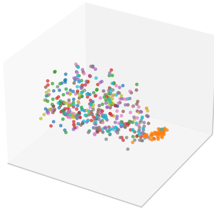
t-SNE
