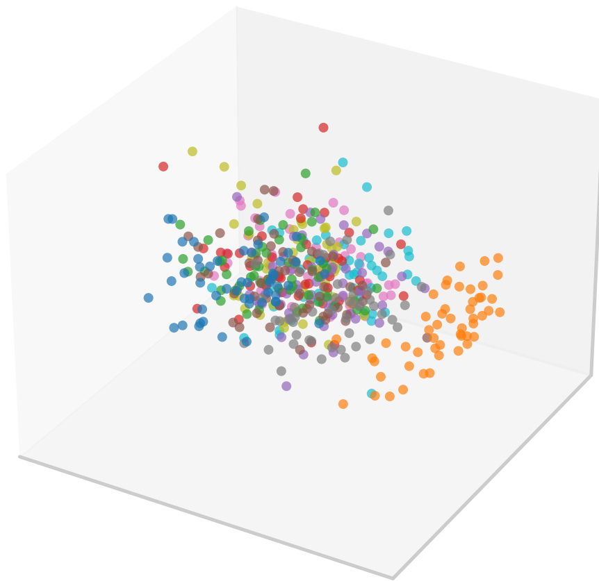
PCA
