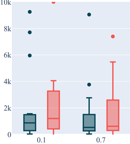
Temperature (Language)
