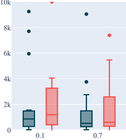
Temperature (Language)
