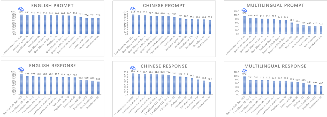
图 1: OpenGuardrails 与现有护栏模型在英语、中文和多语言数据集的提示和响应安全分类基准测试中的平均 F1 分数对比。
