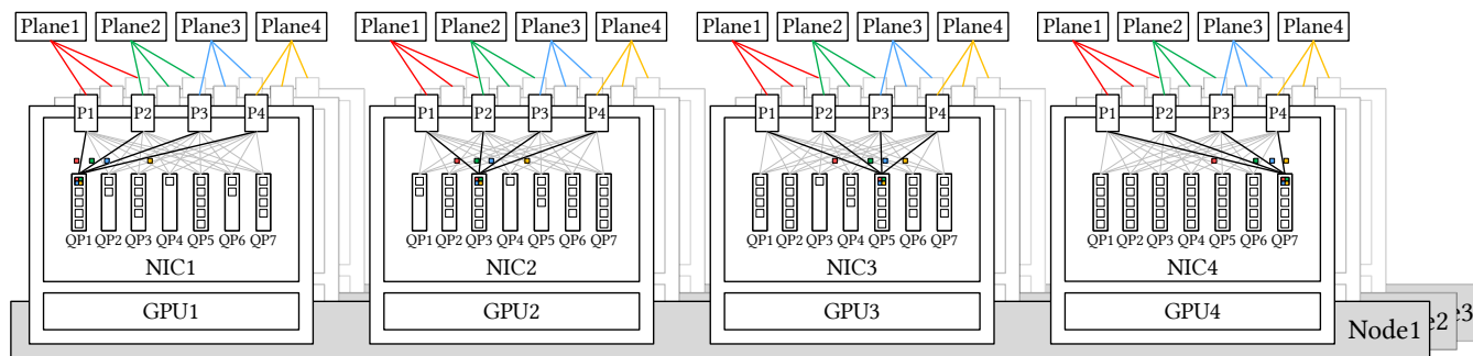
Figure 4: 理想的多平面网络：每个网卡配备多个物理端口，每个端口连接到不同的网络平面。单个队列对（QP）可以同时利用所有可用端口发送和接收数据包，这需要网卡原生支持乱序放置。
