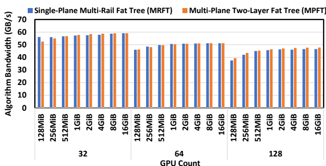
Figure 5: MRFT 和 MPFT 网络在 32 至 128 个 GPU 上的 NCCL all-to-all 性能。
