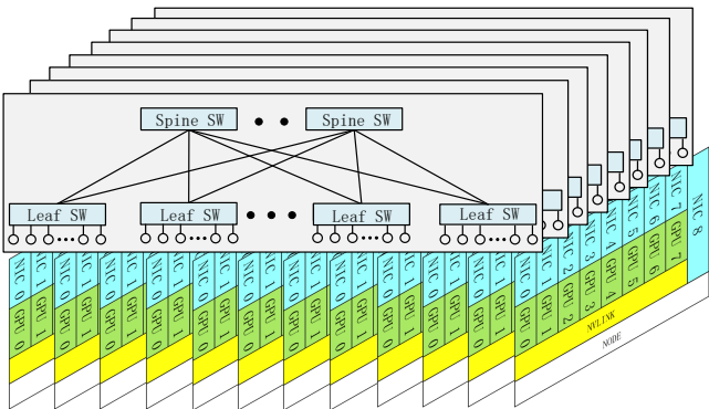
Figure 3: 八平面双层胖树横向扩展网络: 每个 GPU 和 IB 网卡对属于一个网络平面。跨平面流量必须使用另一个网卡以及 PCIe 或 NVLink 进行节点内转发。
