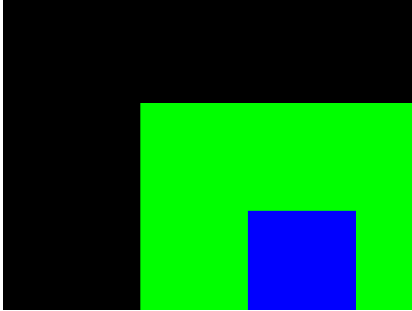
Figura 9 – Reconstituição do defeito de calibração (versão 3.0), obtida executando o próprio gerar_imagem_grade_cores — o mesmo pipeline de renderização de produção — com os parâmetros provisórios de projetor então usados em modo real, apenas para simulação ( f_x = f_y = 500 , c_x = 320 , c_y = 240 , \mathbf{t}_{\text{ext}} = (0, 0, 1)^T ): apenas uma fração da janela é preenchida pela malha, o restante permanece preto. Não é a captura de tela original do incidente de campo, que não foi preservada — é uma reprodução fiel do mecanismo do defeito a partir dos parâmetros documentados na versão 3.0 do código.
