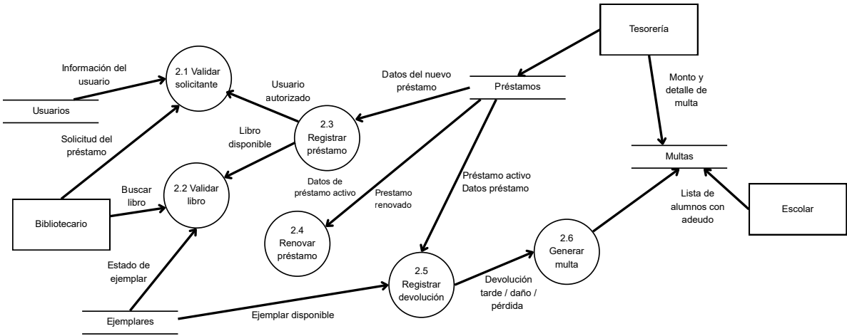
DFD 2 - Gestión de Préstamos y Devoluciones.
