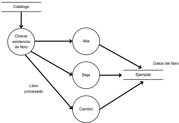
DFD 1 - Gestión de Libros.
