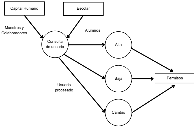
DFD 1 - Gestión de Usuarios.
