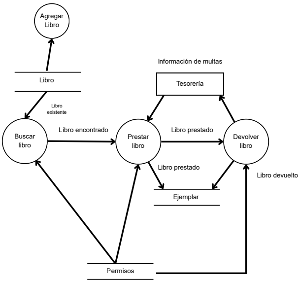
DFD 1 - General.
