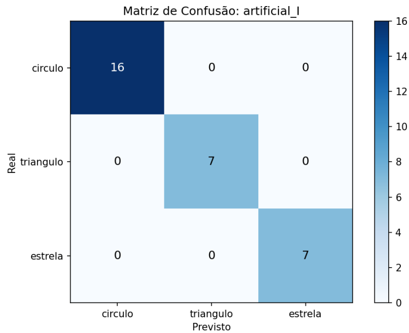
Figura 4: Matrix de confusão — Artificial I.
