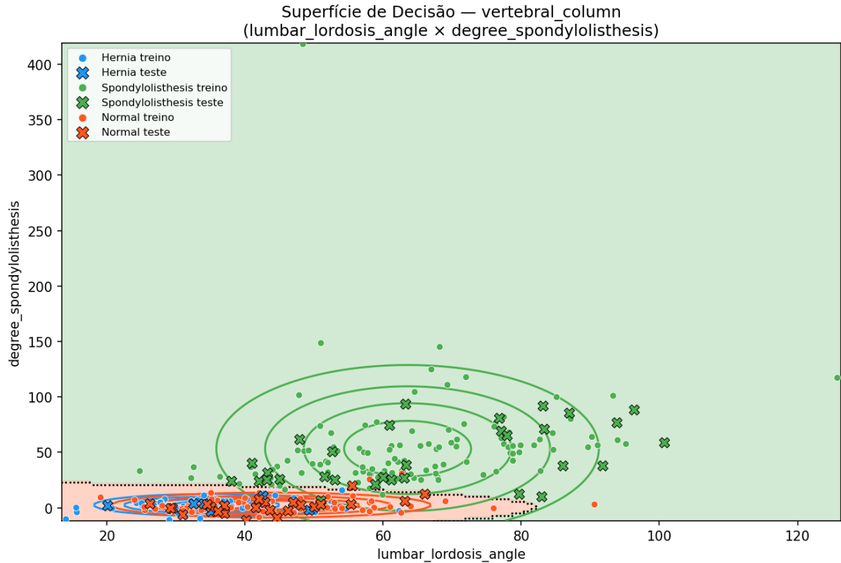
Figura 7: Superfície de decisão — Vertebral Column.
