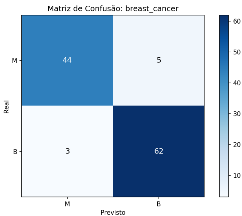
Figura 3: Matriz de confusão — Breast Cancer.
