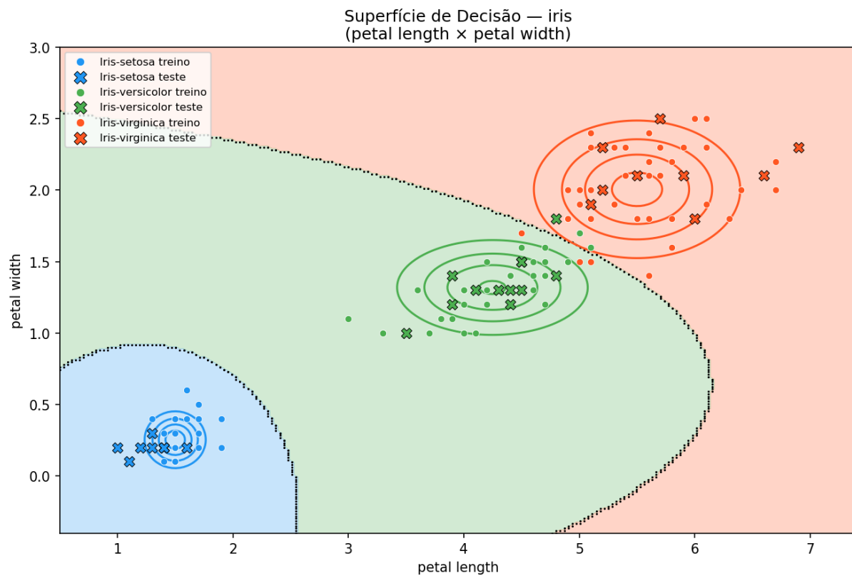
Figura 5: Superfície de decisão — Íris
