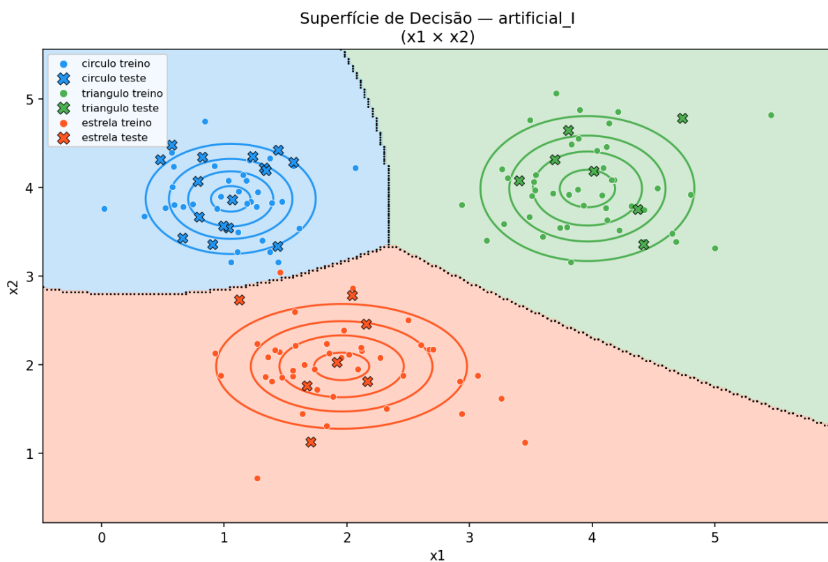
Figura 6: Superfície de decisão — Artificial I
