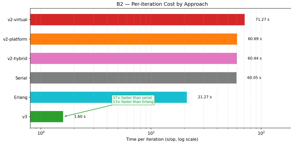
Figure 13: Custo por iteração (B2) em escala logarítmica. As variantes v2 e Serial ficam acima de 60 s/op, dominadas pelo parsing CSV. A v3 cai para 1,60 s/op (37× mais rápida) ao eliminar o I/O das iterações. Erlang fica em 21,27 s/op ( \approx 13\times acima da v3) pelo custo aritmético da BEAM sem vetorização SIMD.
