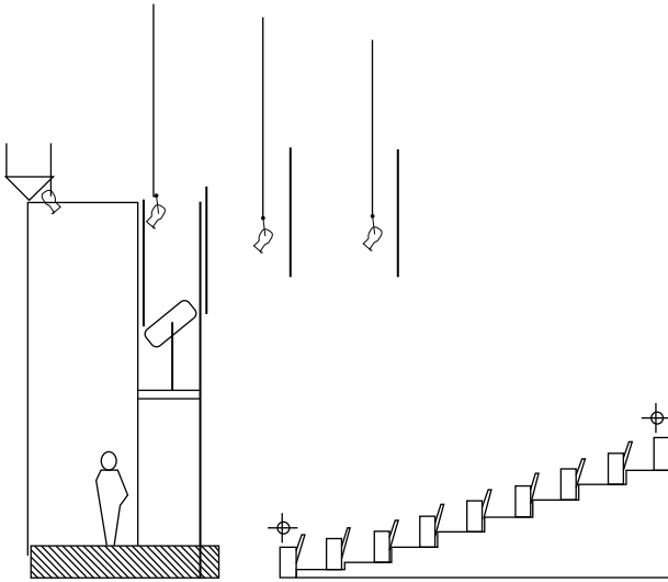
قطاع تقني من المشهد والفضاء المخصّص للجمهور.
