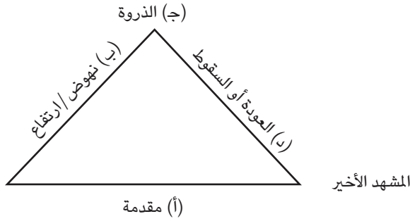
شكل ٤-١: مثلث فرايتاج.
