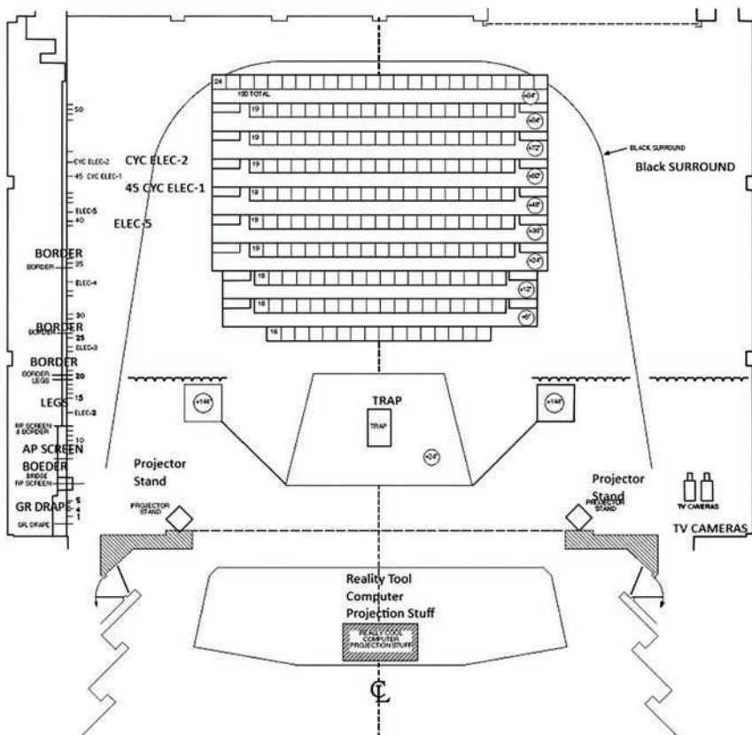
خريطة تقنية للمسرح وللفضاء المخصص للجمهور.
