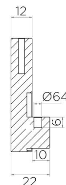
трSL-2912-VN Тримач для труби, бічний (пара),
