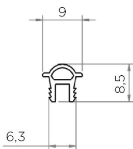
трG-2912 (A10.271-F) Ущільнювач для гардеробної труби, 3000 мм
