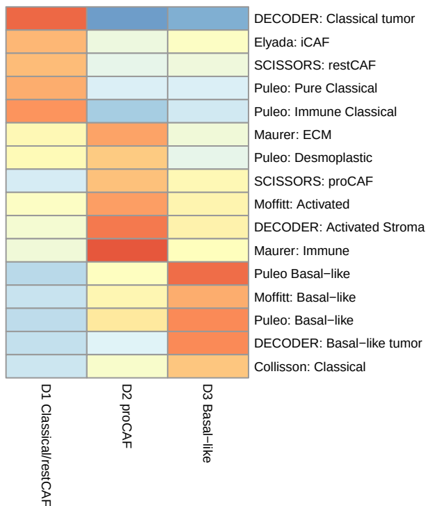
DeSurv
