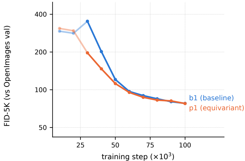
DiT-S/2 (33M)
