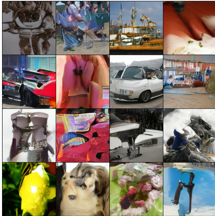
photometric-equivariant (p1)
