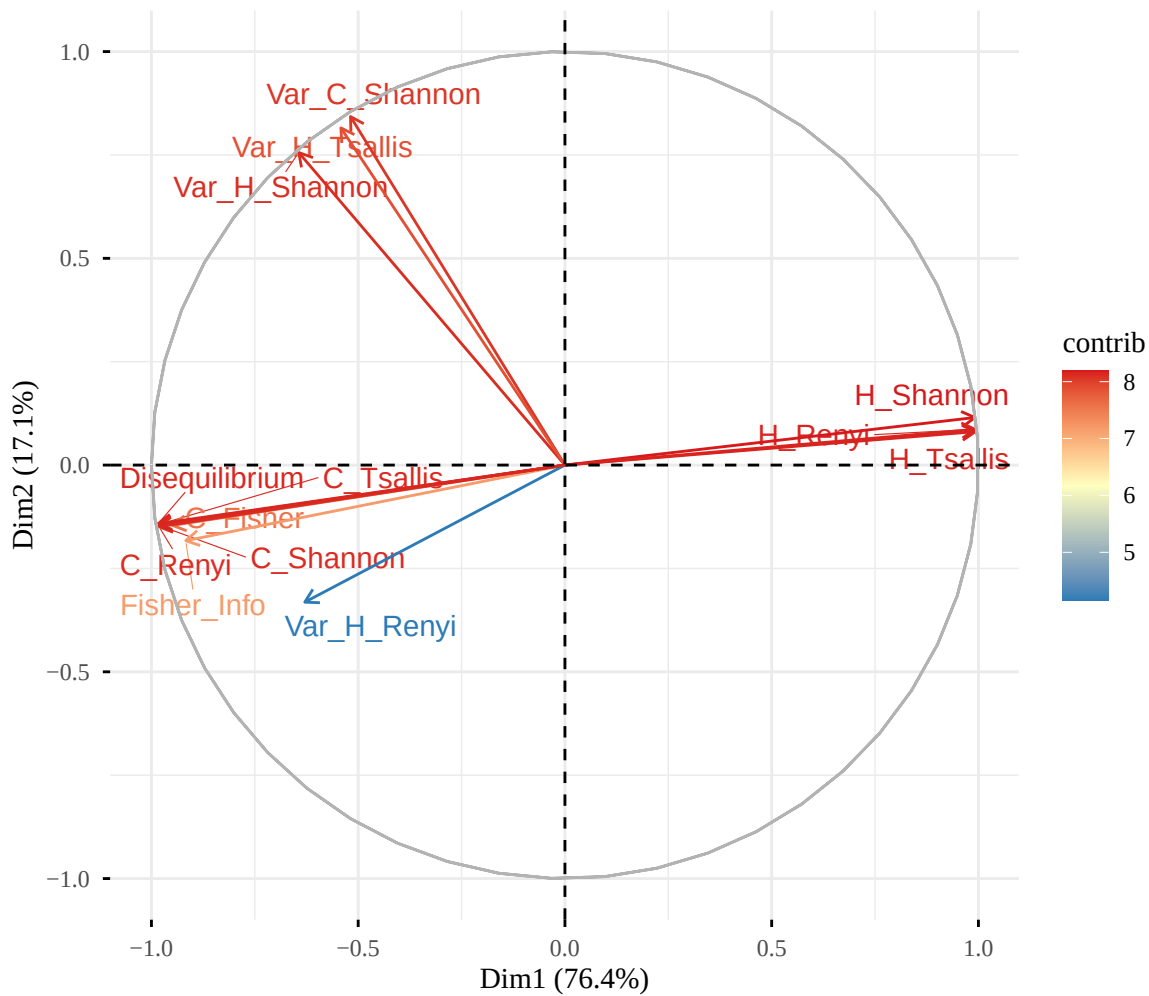
PCA variable loadings (PC1 vs PC2)
