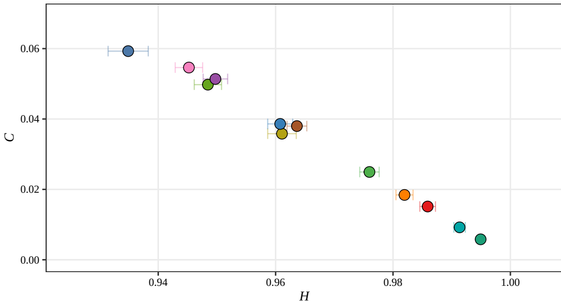
Rényi H-C Plane, D = 5 (RSAM, 2013)
