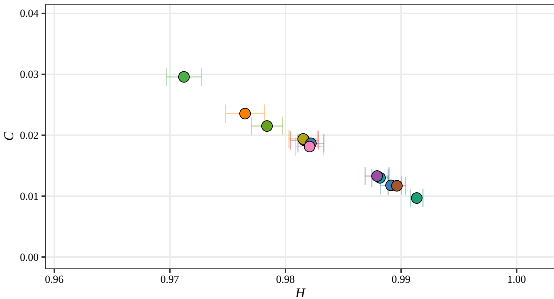
Rényi H-C Plane, D = 5 (RSAM, 2017)
