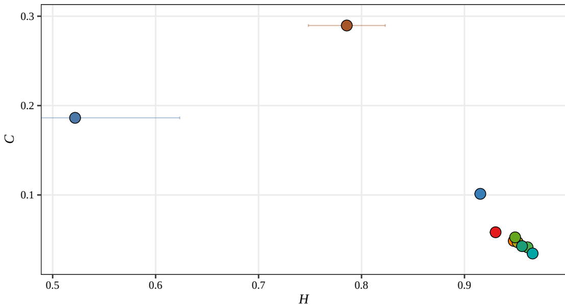
Rényi H-C Plane, D = 5 (RSAM, 2022)
