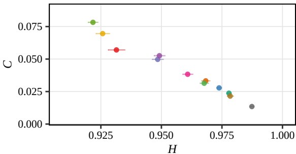
Renyi, D = 5 (RSAM, Apr)
