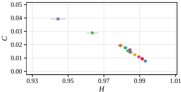
Renyi, D = 5 (Displacement, Feb)
