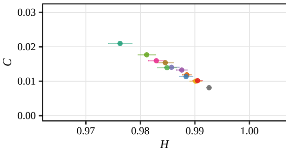
Renyi, D = 5 (Displacement, Jul)
