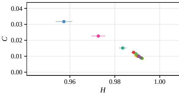
Renyi, D = 5 (Displacement, Jun)
