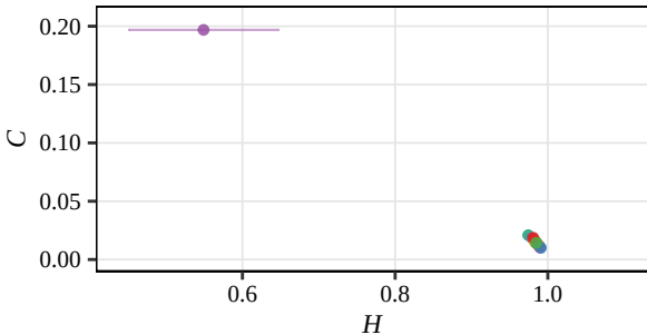
Renyi, D = 5 (Displacement, Sep)
