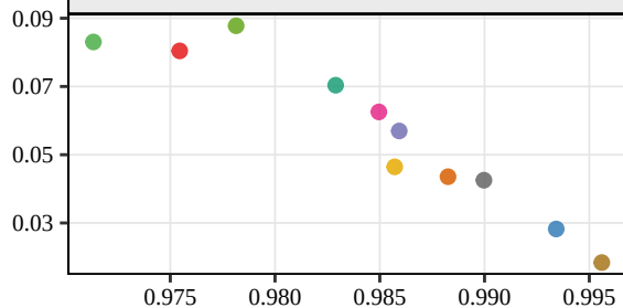
Tsallis
