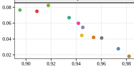
Renyi
