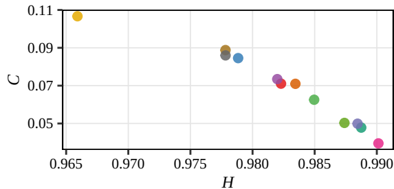
Tsallis
