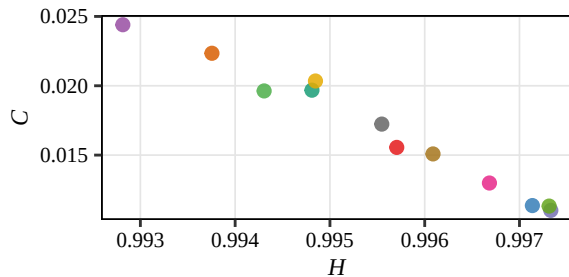
Tsallis
