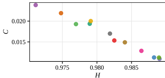
Renyi
