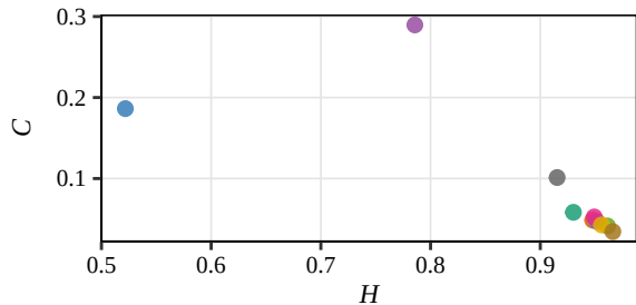
Renyi
