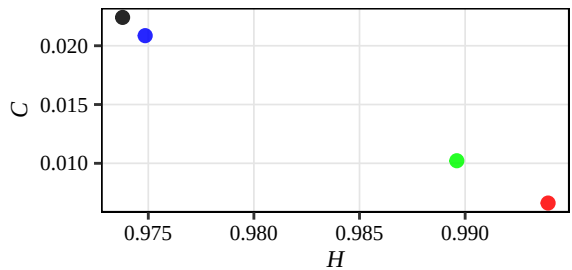
Renyi
