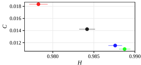
Renyi
