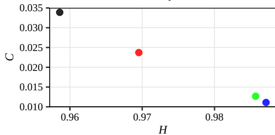
Renyi
