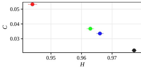
Renyi
