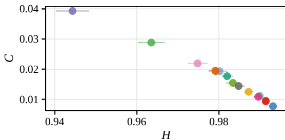
Renyi
