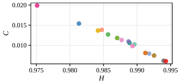
Renyi
