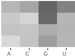
TadA-GFPNb
