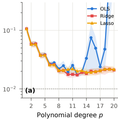
10-fold CV MSE (best \lambda )
