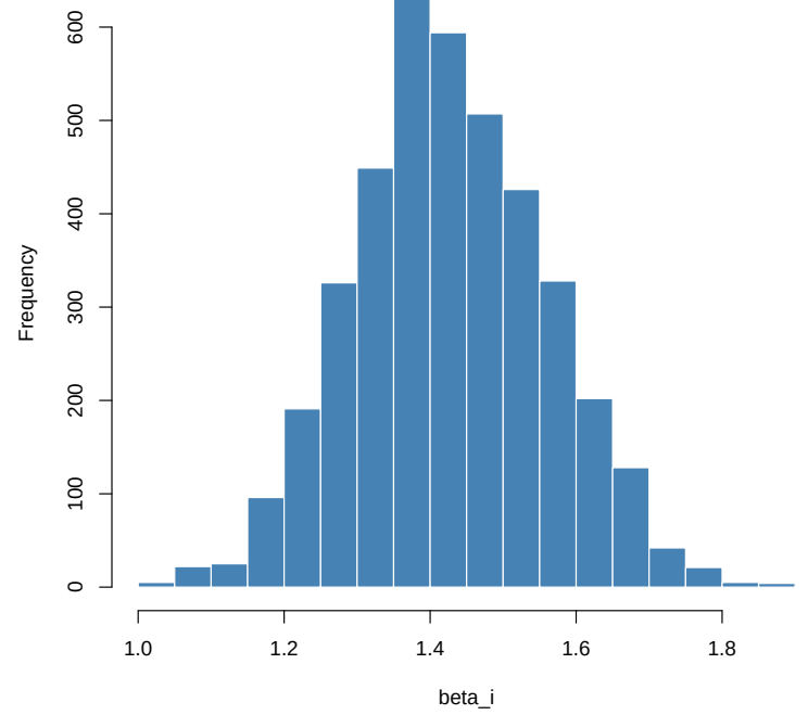
Posterior histogram for \beta_i
