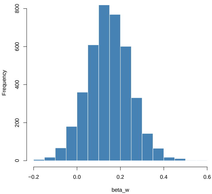
Posterior histogram for \beta_w
