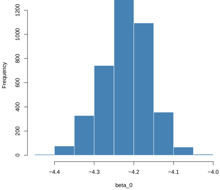
Posterior histogram for \beta_0
