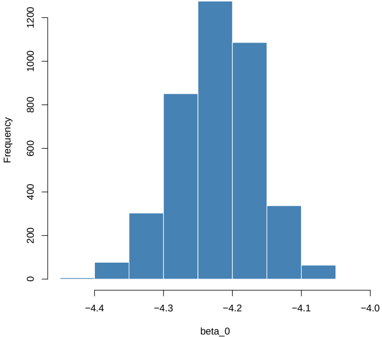
Posterior histogram for beta_0
