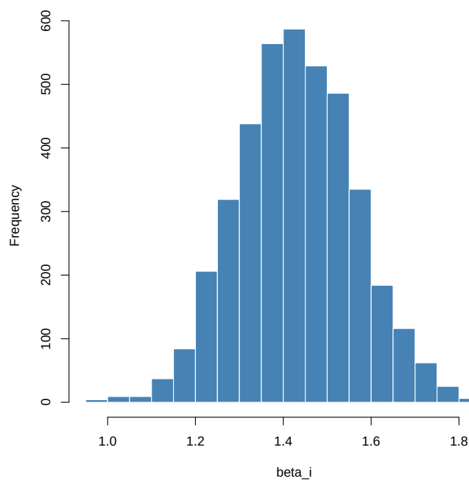
Posterior histogram for beta_i
