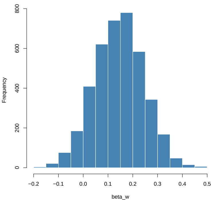
Posterior histogram for beta_w
