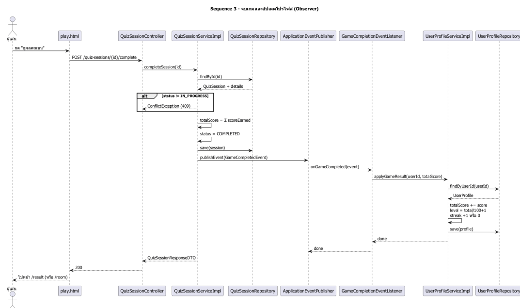
ภาพที่ 8 Sequence Diagram การจบเกมและอัปเดตโปรไฟล์ (Observer)
