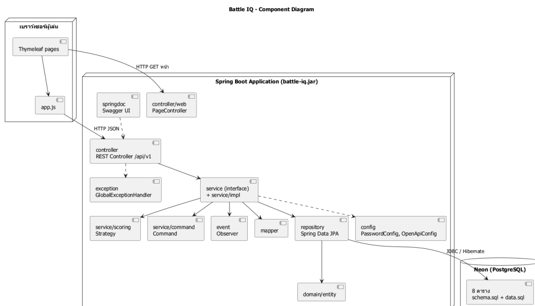
ภาพที่ 3 Component Diagram
