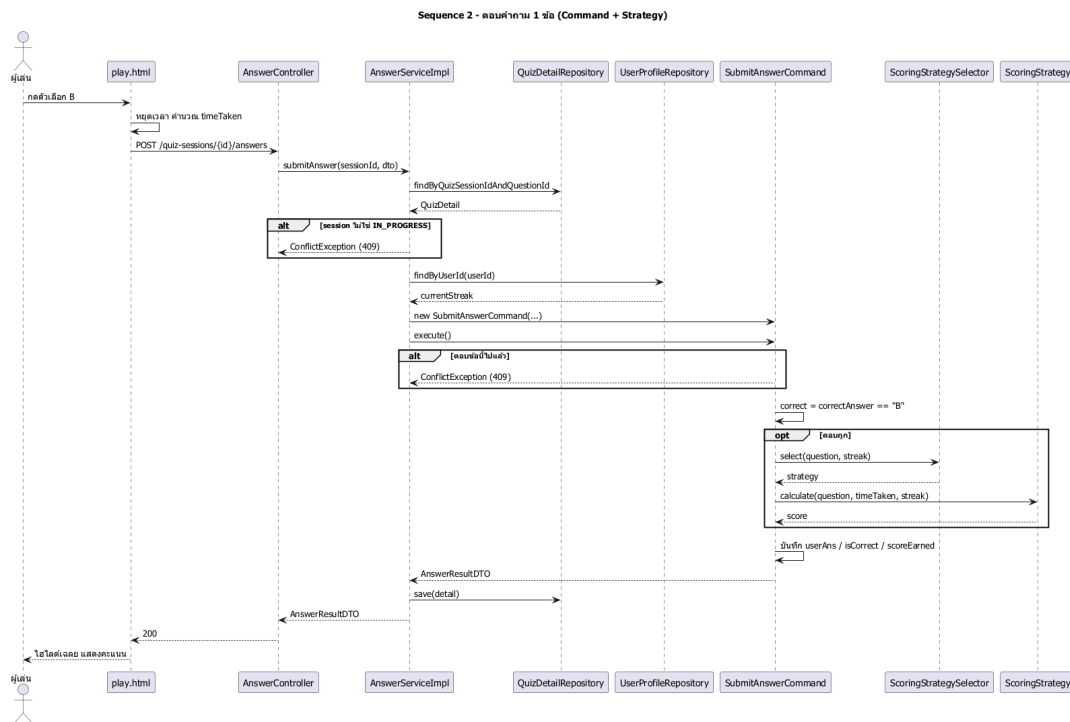
ภาพที่ 7 Sequence Diagram การตอบคำถาม 1 ข้อ (Command และ Strategy)
