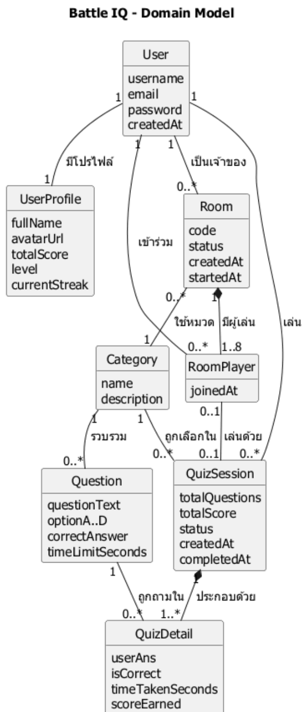
ภาพที่ 2 Domain Model ของระบบ
