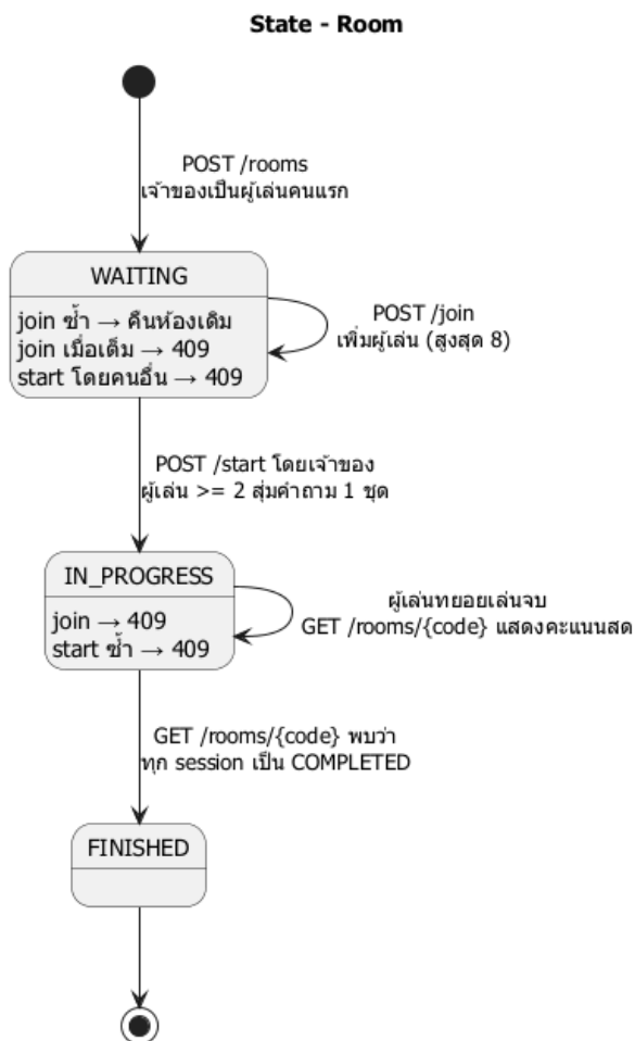
ภาพที่ 13 State Diagram ของ Room
