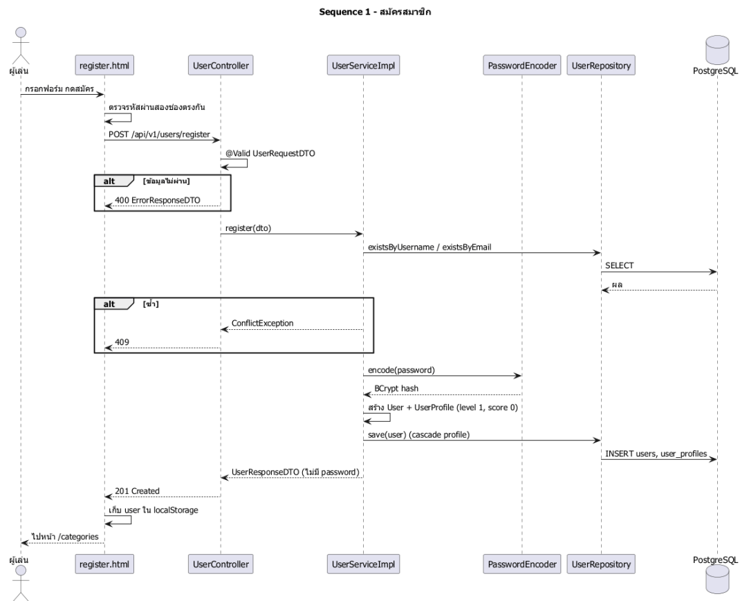
ภาพที่ 6 Sequence Diagram การสมัครสมาชิก
