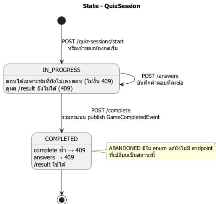
ภาพที่ 12 State Diagram ของ QuizSession
