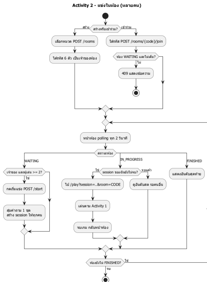
ภาพที่ 11 Activity Diagram การแข่งในห้อง
