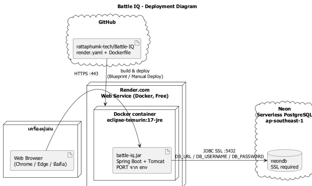
ภาพที่ 4 Deployment Diagram
