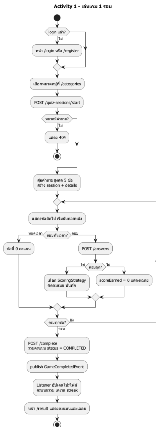
ภาพที่ 10 Activity Diagram การเล่นเกม 1 รอบ
