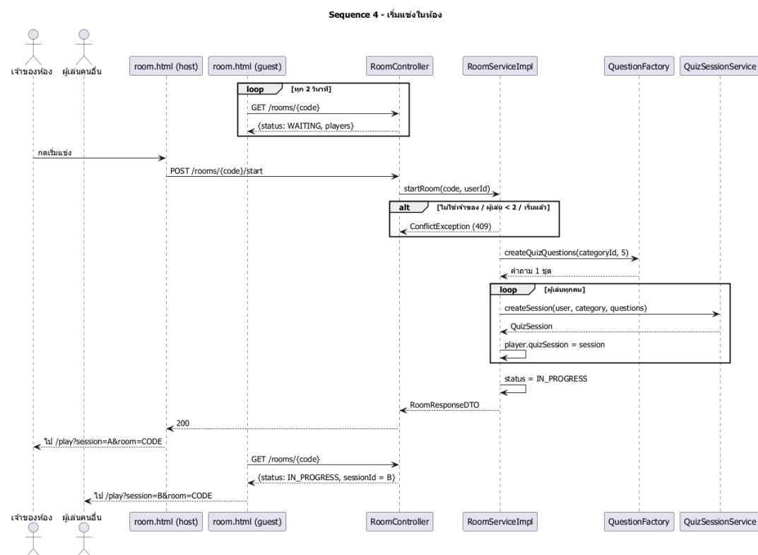
ภาพที่ 9 Sequence Diagram การเริ่มแข่งในห้อง
